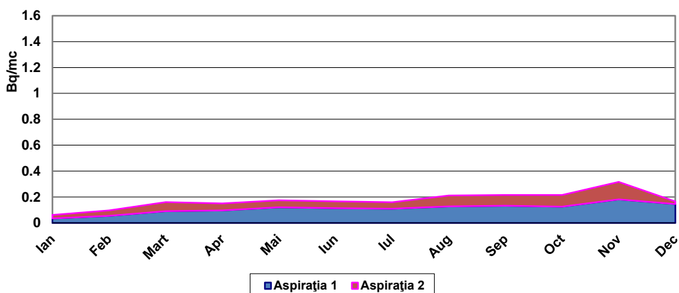
Variația activității specifice mediei lunare a toronului din atmosferă în funcție de variația diurnă
