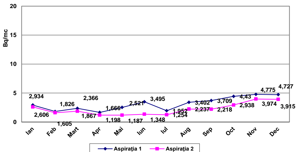
Fig. IX.1.1.1.3. Evoluția mediilor lunare ale radonului în aer
