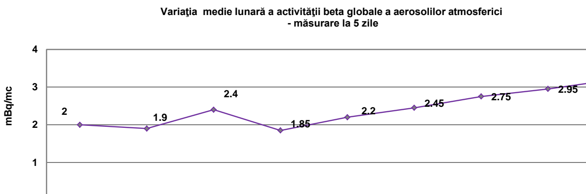
Fig. IX.1.1.1.5 Evoluția mediilor lunare a activității beta globale a aerosolilor atmosferici - măsurare la 5 zile
