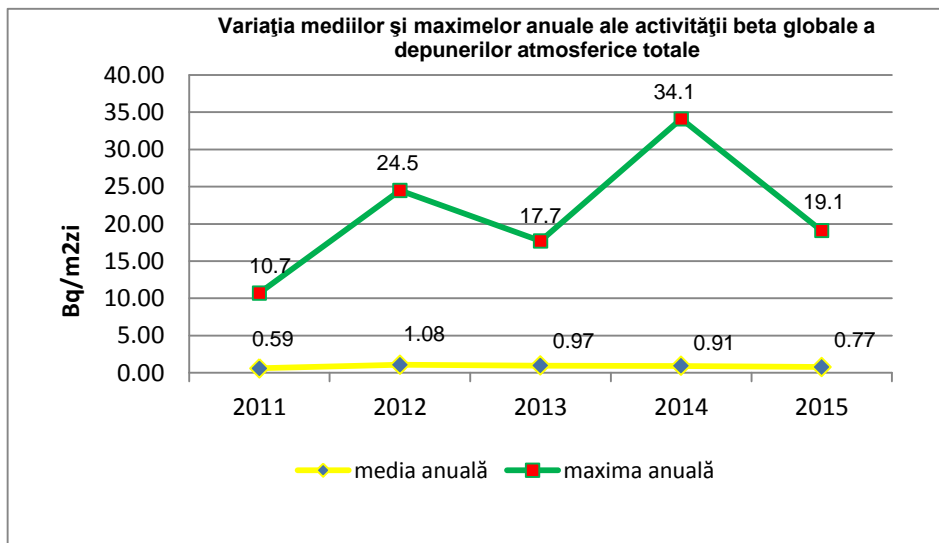
Fig. IX.1.1.2.2. Variația anuală a activității specifice beta globale pentru depuneri atmosferice uscate și umede
