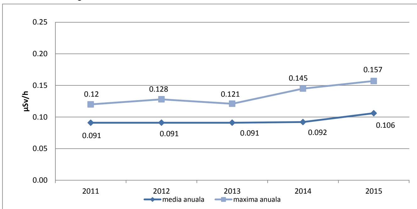
Fig. IX.1.1.2.a. Evoluția anuală a debitului dozei gamma în aer
