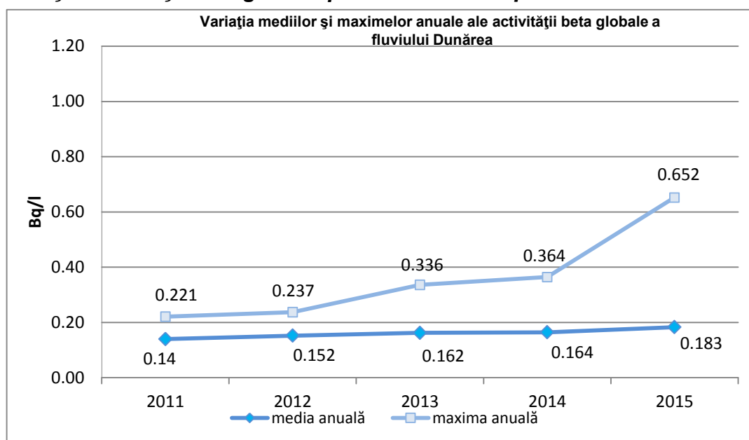
Fig. IX.1.2.1.2. Evoluția anuală a activității beta globale pentru Dunăre
