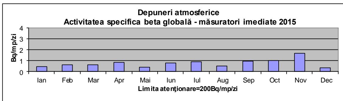
Fig. IX.1.1.2.1. Variația lunară a activității specifice beta globale pentru depuneri atmosferice uscate și umede
