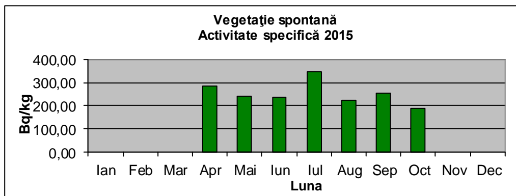
Fig.I X.1.4.1. Evoluția lunară a activității beta globale pentru vegetație
