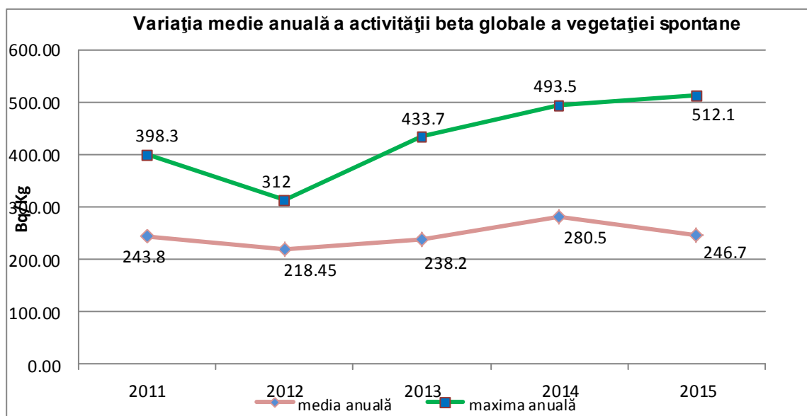
Fig. IX.1.4.2. Evoluția anuală a activității beta globale pentru vegetație
