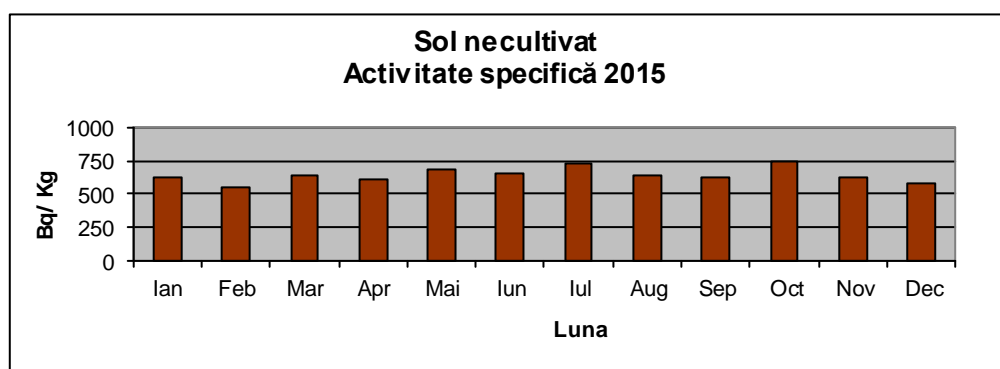
Fig.IX.1.3.1. Evoluția lunară a activității beta-globale pentru sol necultivat
