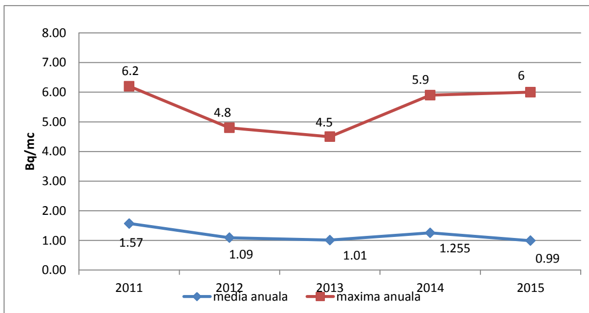
Fig. IX.1.1.1.2. Variația mediilor anuale ale activității specifice beta globale pentru aerosoli atmosferici
