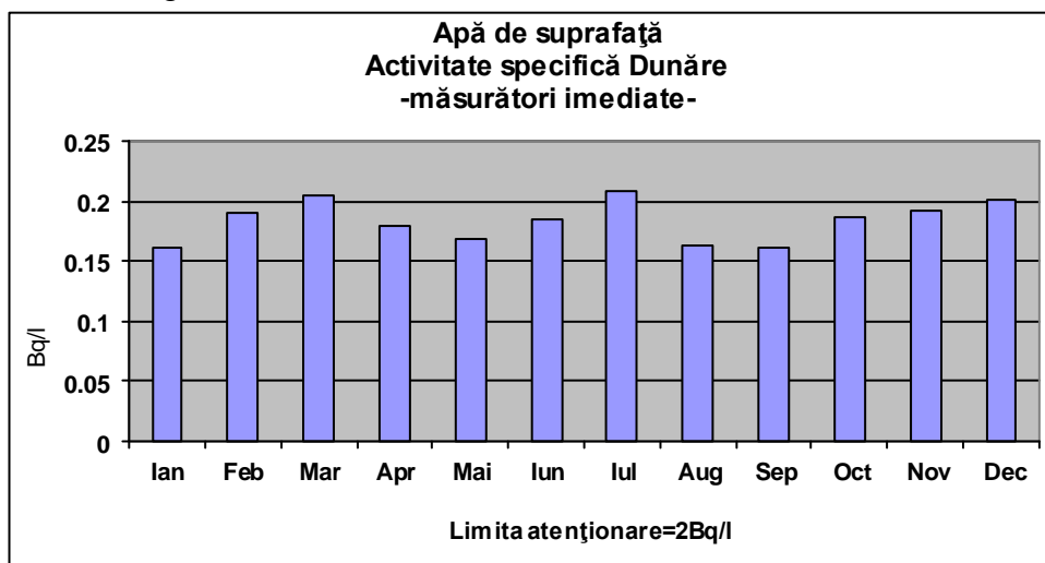
Fig. IX.1.2.1.1. Evoluția lunară a activității beta globale pentru Dunăre
