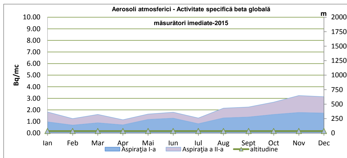
Fig. IX.1.1.1.1. Variația mediilor lunare ale activității specifice beta globale pentru aerosoli atmosferici
