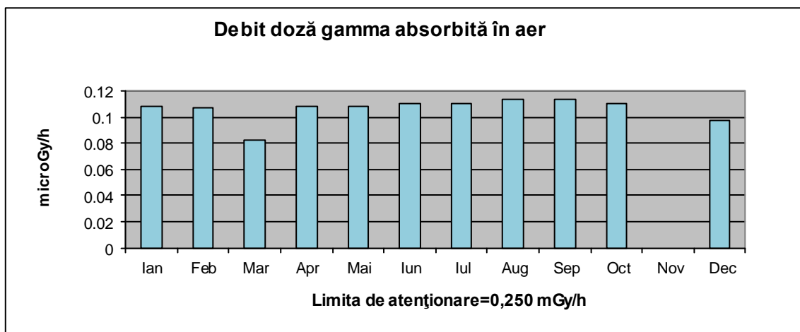
Fig.I X.1.1.1.a. Evoluția lunară a debitului dozei gamma în aer
