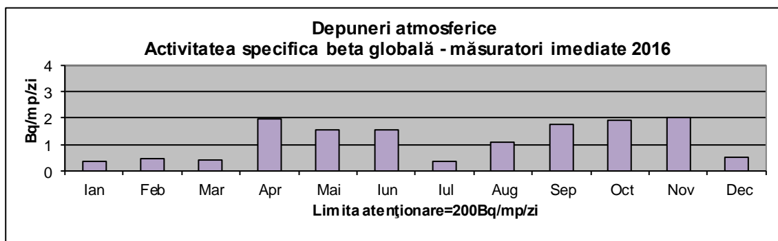
Fig. IX.1.1.2.1. Variația lunară a activității specifice beta globale pentru depunerii atmosferice uscate și umede
