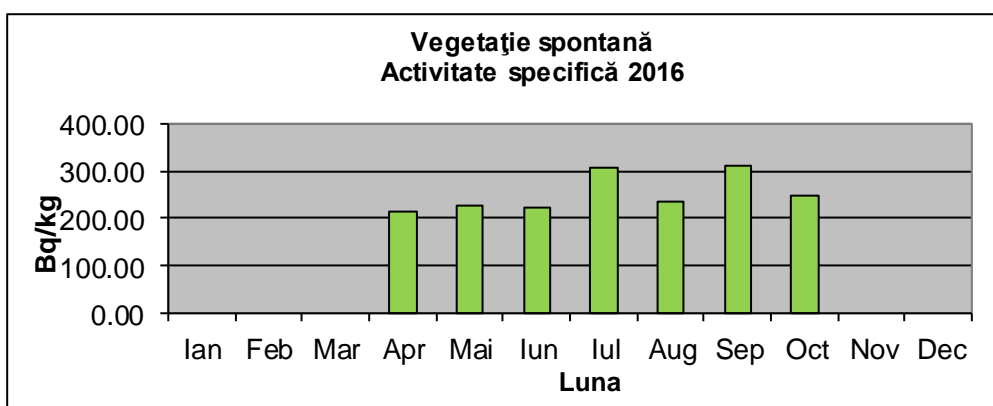
Fig.I X.1.4.1. Evoluția lunară a activității beta globale pentru vegetație
