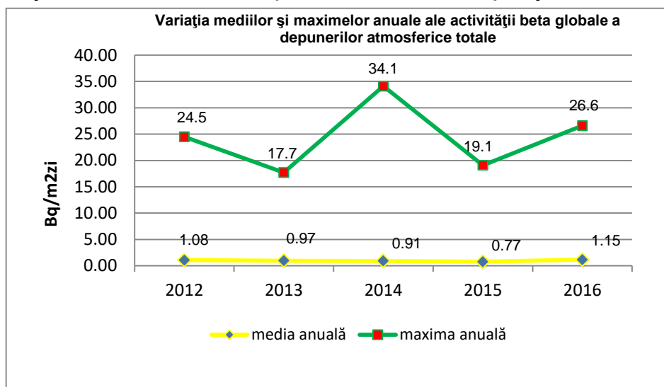
Fig. IX.1.1.2.2. Variația anuală a activității specifice beta globale pentru depunerii atmosferice uscate și umede
