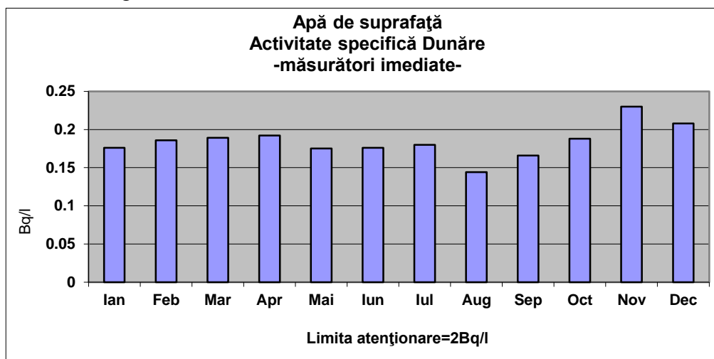
Fig. IX.1.2.1.1. Evoluția lunară a activității beta globale pentru Dunăre
