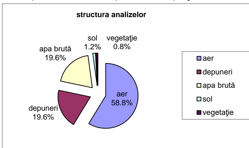
Fig. IX.1.1. Distribuția procentuală de analize pe tipuri de probe prelevate în anul 2016
