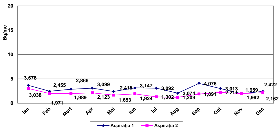
Fig. IX.1.1.1.3. Evoluția mediilor lunare ale radonului în aer
