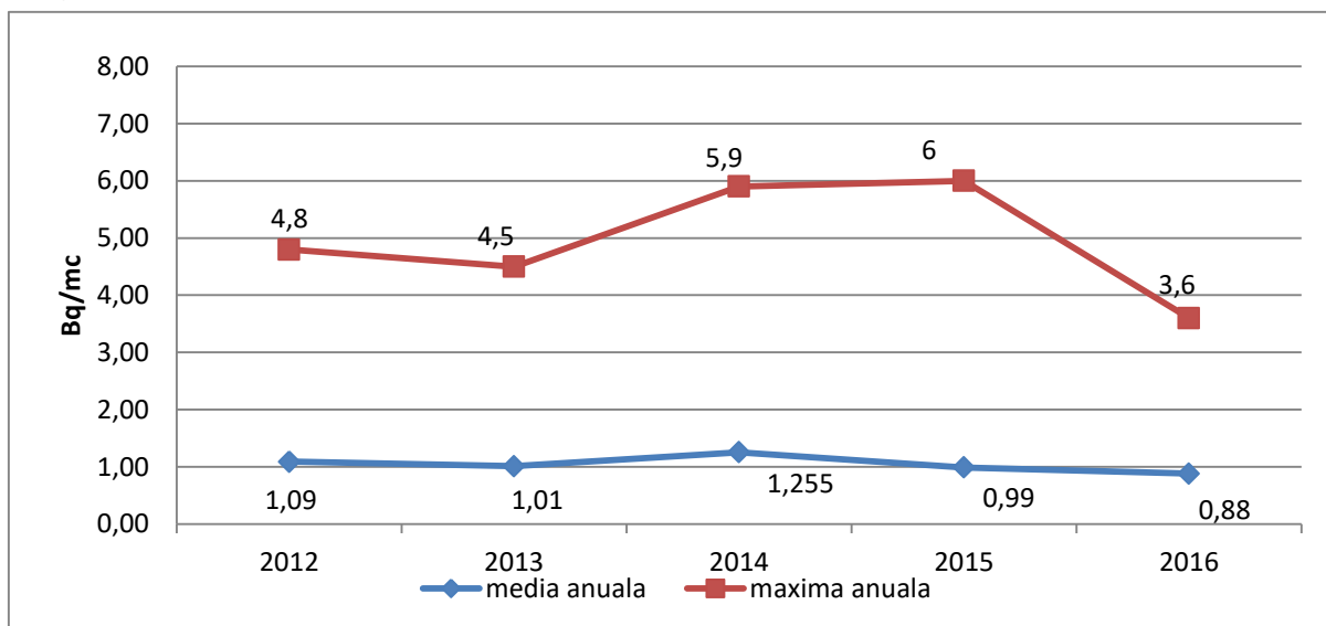
Fig. IX.1.1.1.2. Variația mediilor anuale ale activității specifice beta globale pentru aerosoli atmosferici
