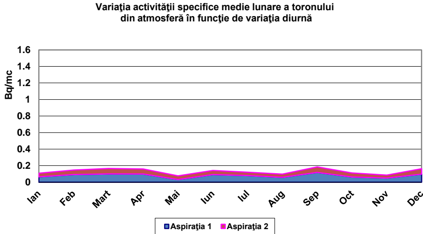
Fig.IX.1.1.1.4. Evoluția mediilor lunare ale toronului în aer
