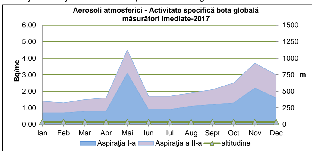
Fig. IX.1.1.1.1. Variația mediilor lunare ale activității specifice beta globale pentru aerosoli atmosferici
