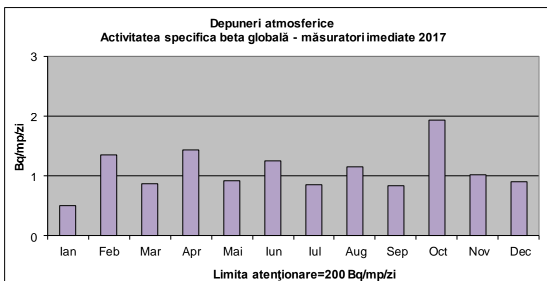
Fig. IX.1.1.2.1. Variația lunară a activității specifice beta globale pentru depuneri atmosferice uscate și umede
