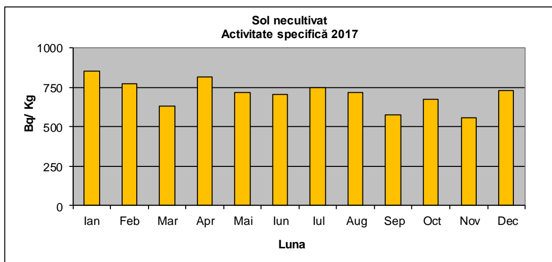
Fig.IX.1.3.1. Evoluția lunară a activității beta-globale pentru sol necultivat
