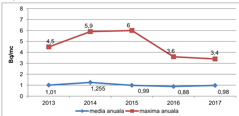
Fig. IX.1.1.1.2. Variația mediilor anuale ale activității specifice beta globale pentru aerosoli atmosferici
