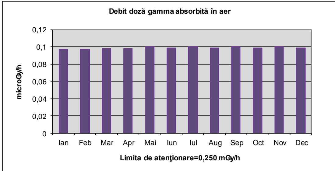
Fig.I X.1.1.1.a. Evoluția lunară a debitului dozei gamma în aer
