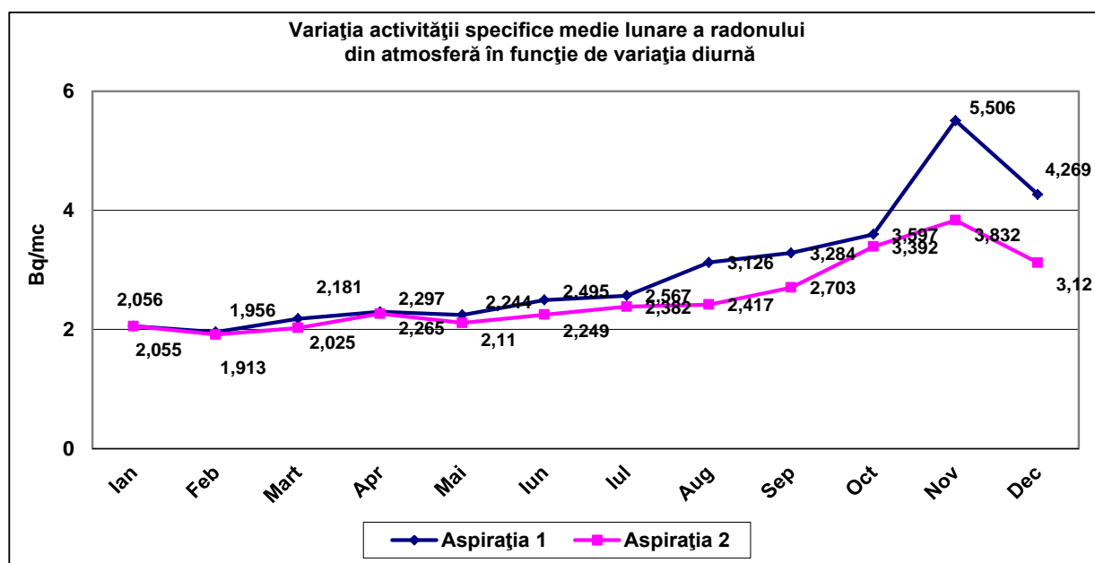
Fig. IX.1.1.1.3. Evoluția mediilor lunare ale radonului în aer
