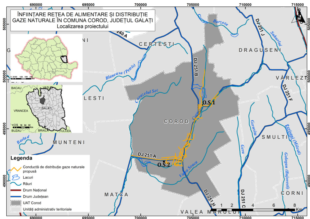
Figura nr. 6: Plan de încadrare în zonă a organizărilor de șantier (UAT Corod)
