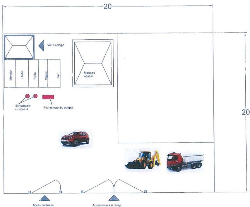
Organizare de șantier – Plan de situație
