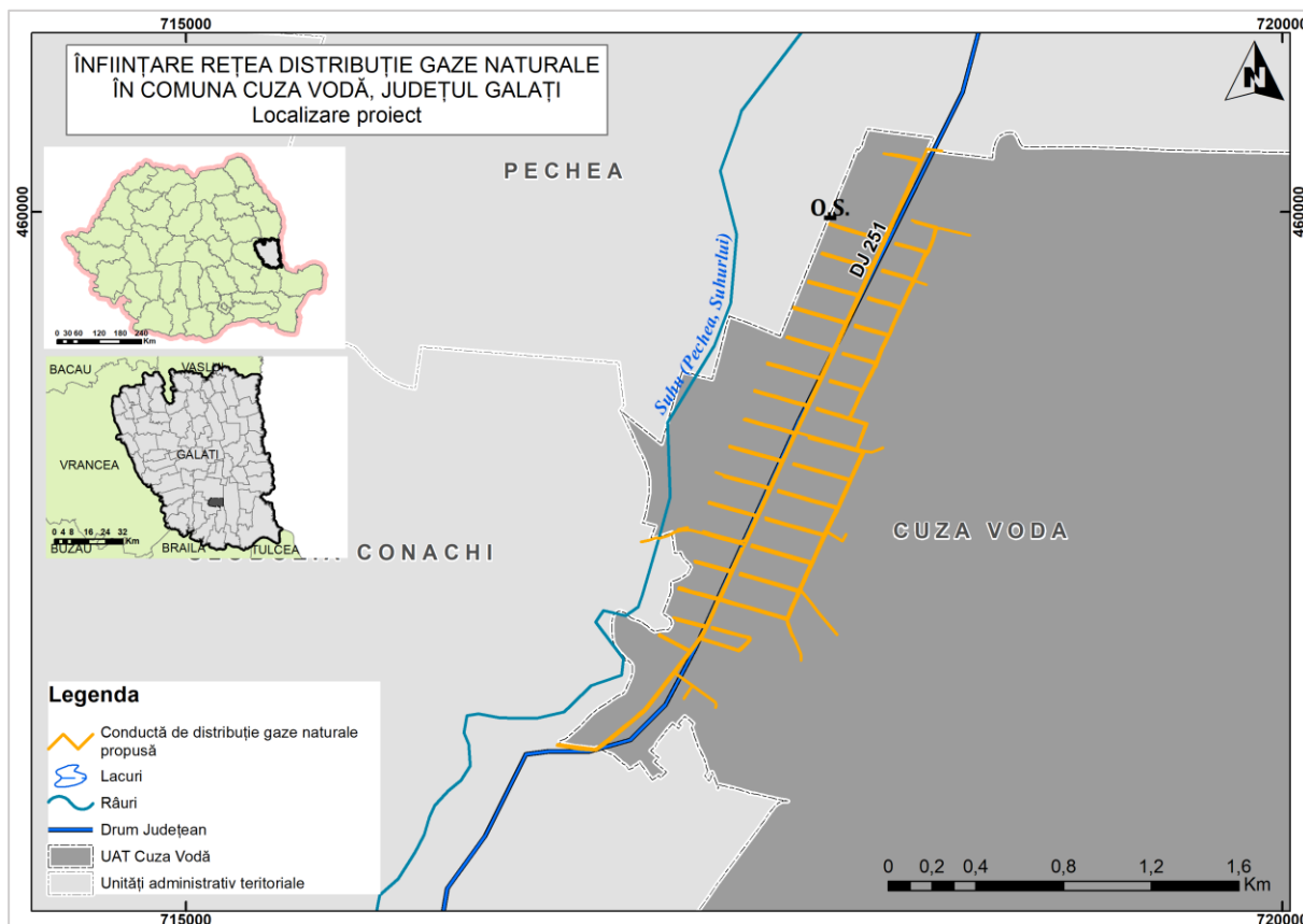
Figura nr. 6: Plan de încadrare în zonă a organizării de șantier - UAT Cuza Vodă
