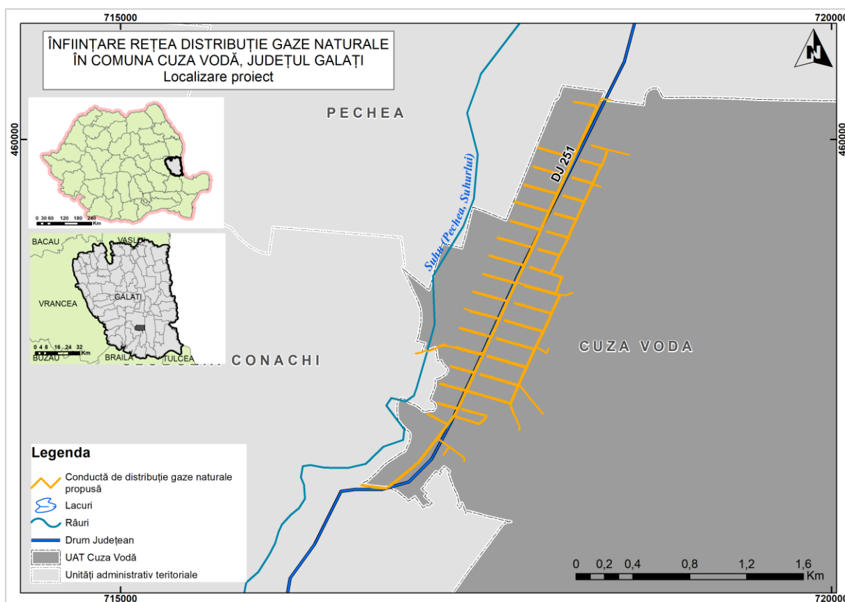
Figura nr. 1: Plan de situație amplasare proiect „Înființare rețea de distribuție gaze naturale în comuna Cuza Vodă, județul Galați”
