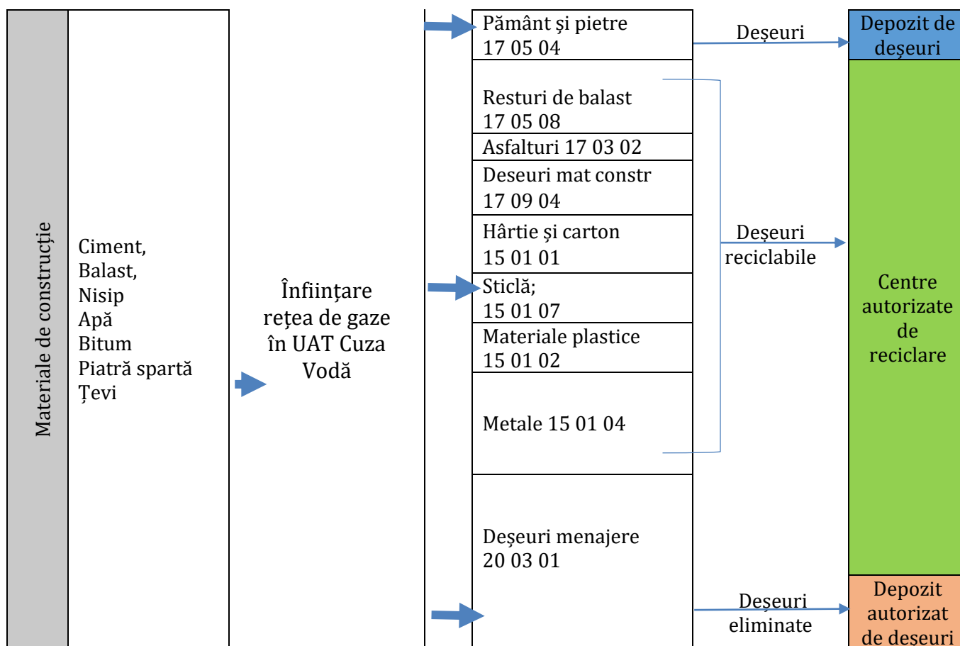
Figura nr. 7: Schema flux de gestionare a deșeurilor
