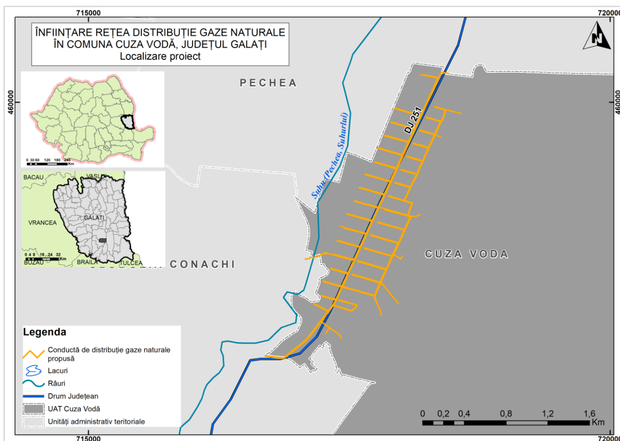
Figura nr. 4: Localizare proiect rețea gaze naturale (comuna Cuza Vodă)
