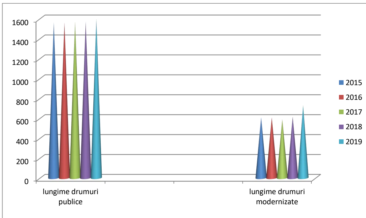
Figura IV 3.2.1. Evoluția lungimii drumurilor publice și a celor modernizate, la nivelul județului Galați, în perioada 2015 – 2019
