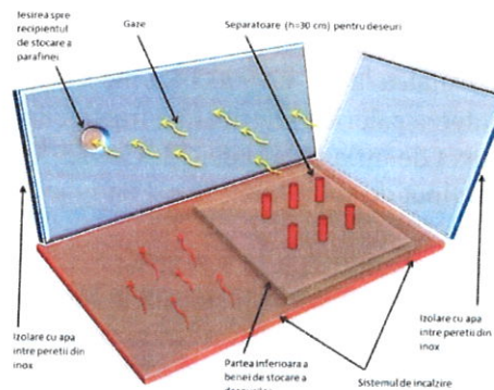
Reactorul de procesare fizico-chimică a deșeurilor
