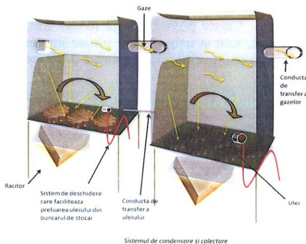
Sistemul de condensare și colectare
