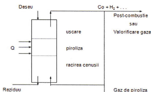
Figura nr. 3 - Piroliza de joasă temperatură
