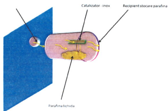
Ilustrație privind catalizarea gazului și colectarea parafinei
