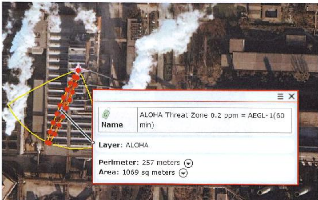
Zona de impact Convertizor nr. 1 – Dioxid de sulf ( \text{SO}_2 ) Galben: 126 m; Perimetru: 257 m; Suprafața: 1069 mp; Conc.: 0,2 ppm = AEGL-1 (60 min)
