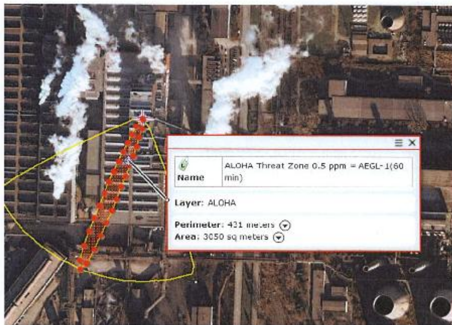
Zona de impact Convertizor nr. 1- Dioxid de azot (NO 2 ) Galben: 213 m; Perimetru: 431 m; Suprafata: 3050 mp; Conc. 0,5 ppm = AEGL-1 (60 min);
