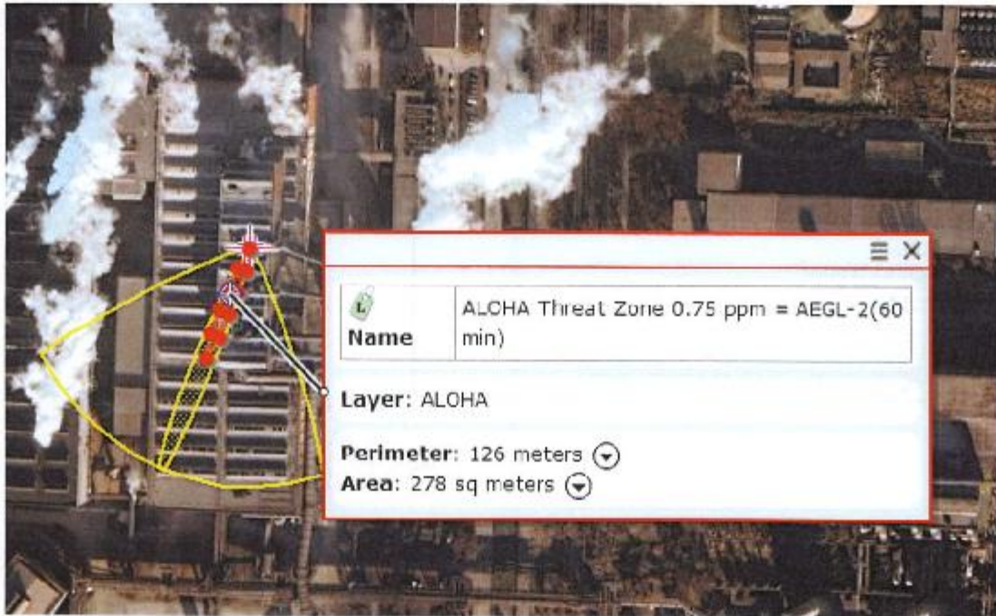
Zona de impact Convertizor nr. 1 – Dioxid de sulf ( \text{SO}_2 ) Portocaliu: 62 m; Perimetru: 126 m; Suprafața: 278 mp; Conc.: 0.75 ppm = AEGL-2 (60 min)
