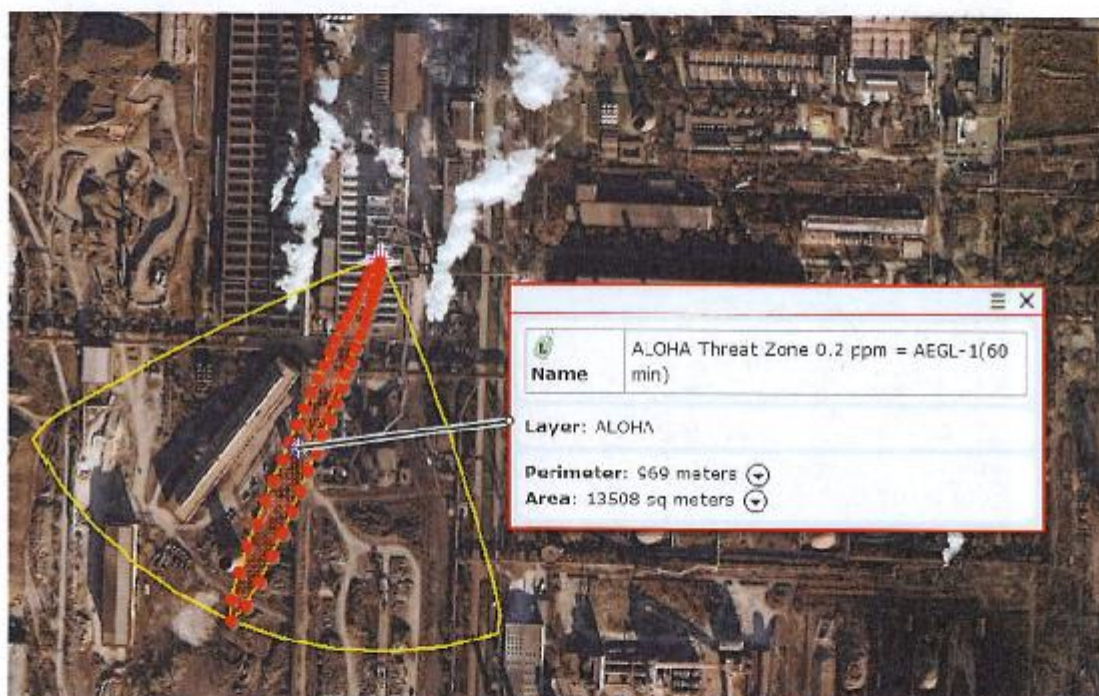
Zona de impact Convertizor nr. 3 – Dioxid de sulf ( \text{SO}_2 ) Galben: 480 m; Perimetru: 969 m; Suprafața: 13508 mp; Conc. 0,2 ppm = AEGL-1 (60 min)
