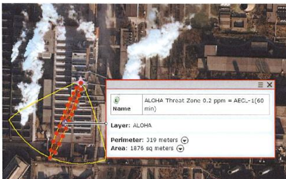
Zona de impact Convertizor nr. 2 – Dioxid de sulf ( \text{SO}_2 ) Galben: 157 m; Perimetru: 319 m; Suprafața: 1876 mp; Conc. 0,2 ppm = AEGL-1 (60 min)
