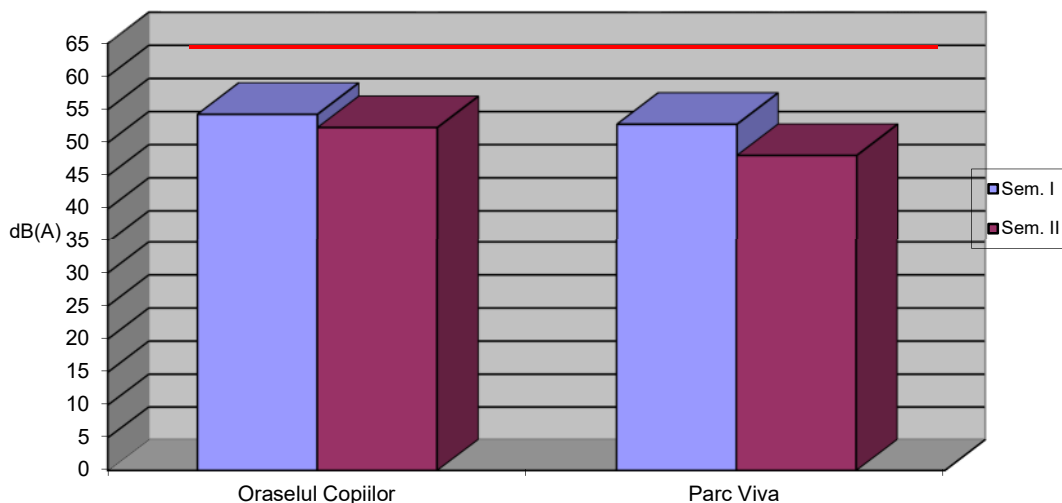
Figura VIII.1.2.1.2. Valori ale nivelului de zgomot echivalent măsurat în parcuri, medii semestriale 2021
